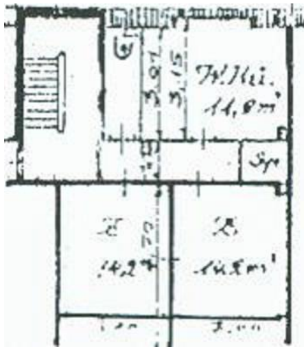
Grundriss Dachgeschoss Gruppenhaus
